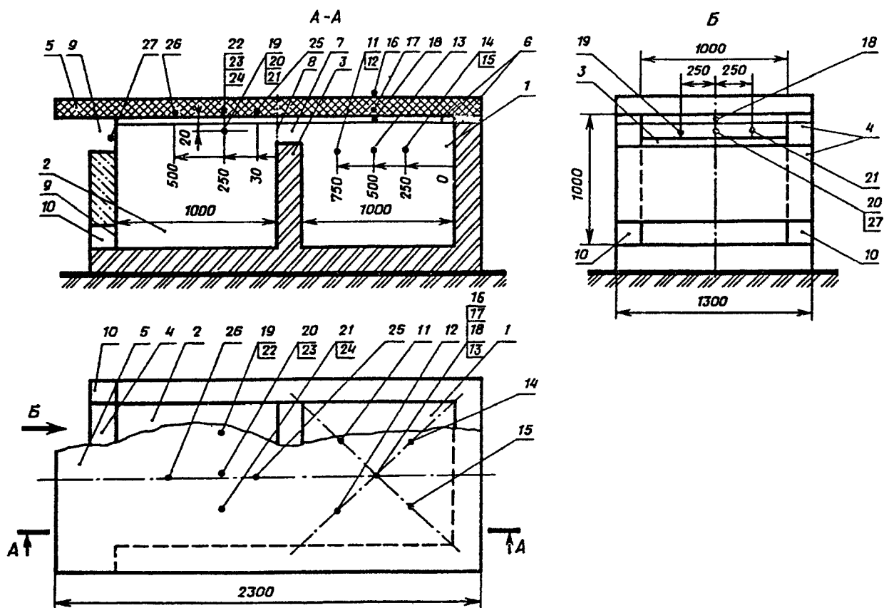
Рисунок 1. Схема печи для испытаний вертикальных конструкций и установки на ней образца конструкции
